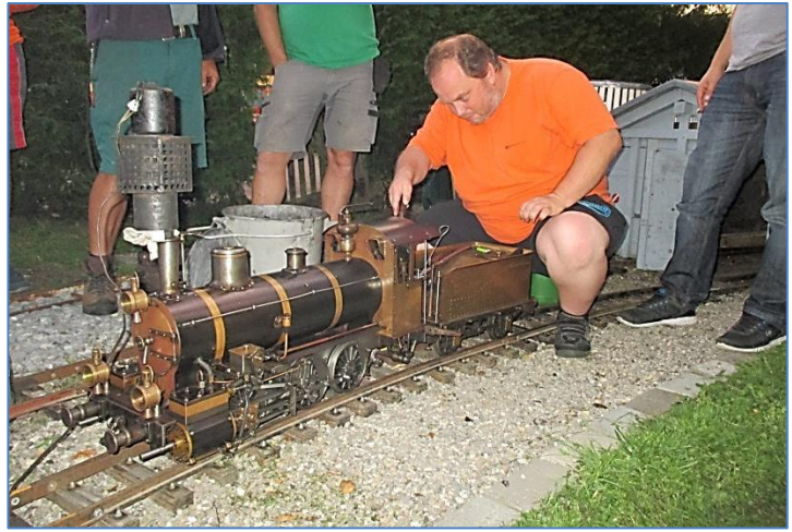
Und bald geht die Fahrt los. Die Lok zieht mühelos 7 Personen auf Wägelchen durch den Garten!
